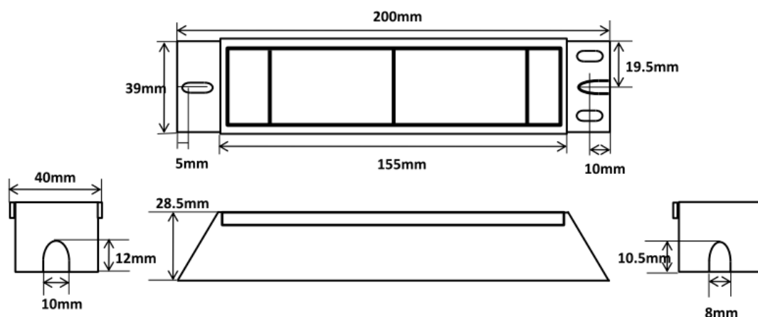
電源ユニット寸法図（図：6）
